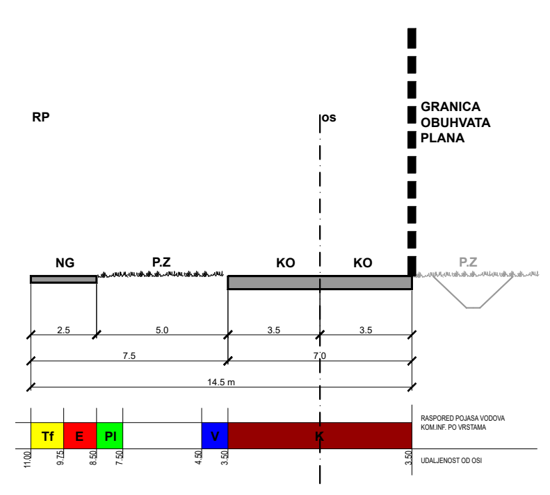
KARAKTERISTIČNI PROFIL PROMETNICE A-A S NAČELIMA RASPOREDA VODOVA KOMUNALNE INFRASTRUKTURE U MJERILU 1:500
