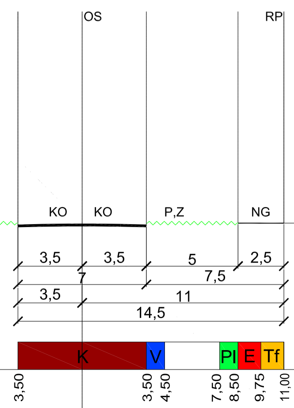
KARAKTERISTIČNI PROFIL PROMETNICE B-B S NAČELIMA RASPOREDA VODOVA KOMUNALNE INFRASTRUKTURE U MJERILU 1:500
